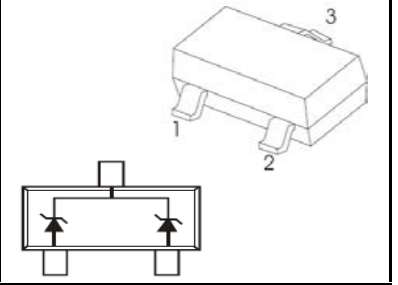
SOT-23
